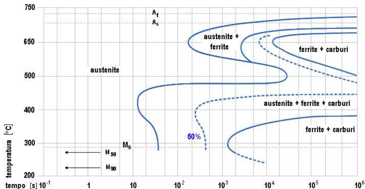
Diagramma di trasformazione isothermico - tempo - temperature
